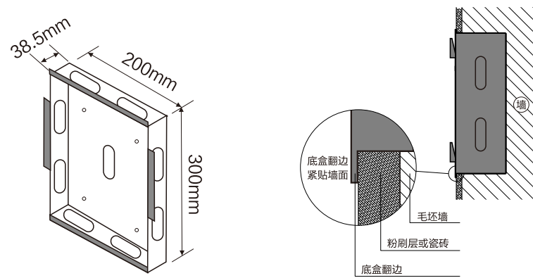
附-- 安装方式示意图（单位mm）：
